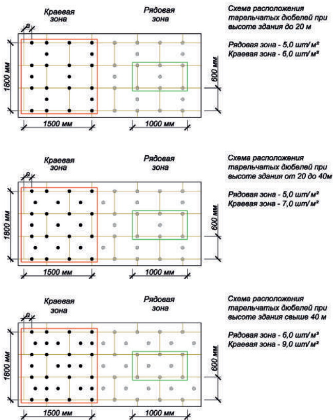
Рис. 13. Рекомендуемая схема расположения тарельчатых дюбелей на плоскости фасада
