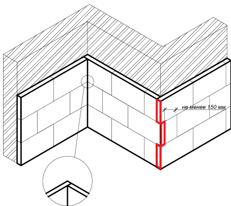
Рис. 9. Схема перевязки плит на внутренних и наружных углах здания
